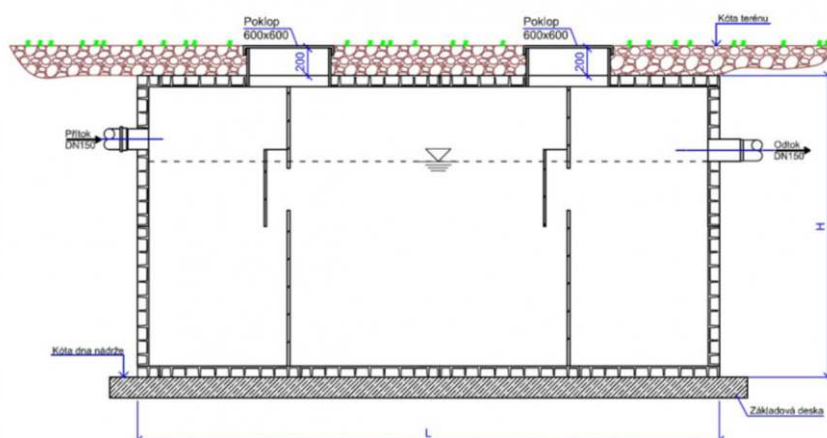
SEPTIKOVÉ NÁDRŽE HRANATÉ - SAMONOSNÉ
