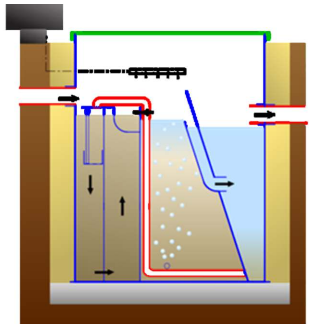
Schéma DČOV zdroj
